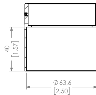
SEZIONE A-A
