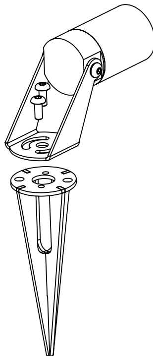
MONTAGGIO ACCESSORIO MOON MARINE
